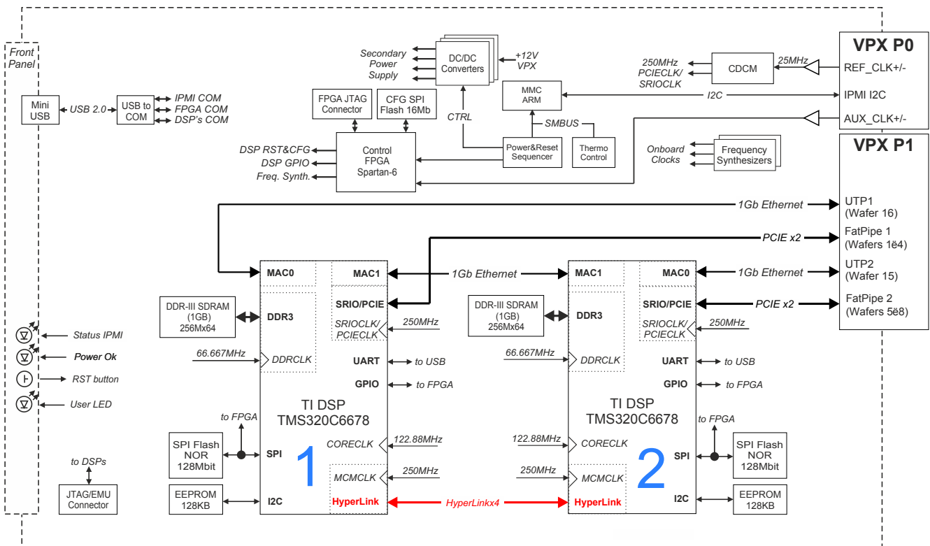
Рисунок 1-1: Структурная схема модуля SVP-405
