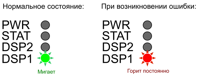
Рисунок 7-2: Светодиоды на передней панели модуля SVR-420
